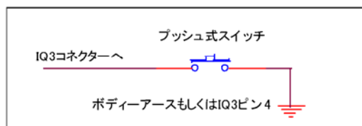
スイッチ配線図
